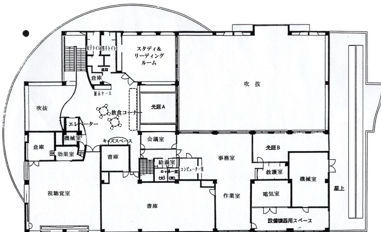
2 階平面図
